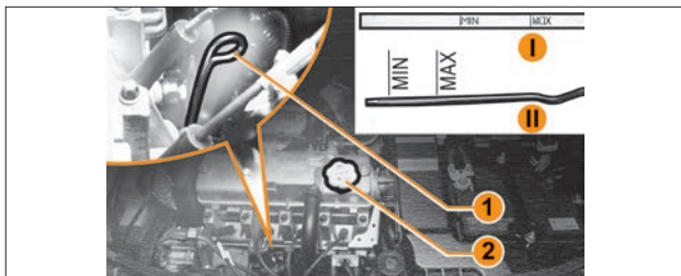
Рис. 6.3.1. Масляный щуп двигателя (в варианном исполнении)
