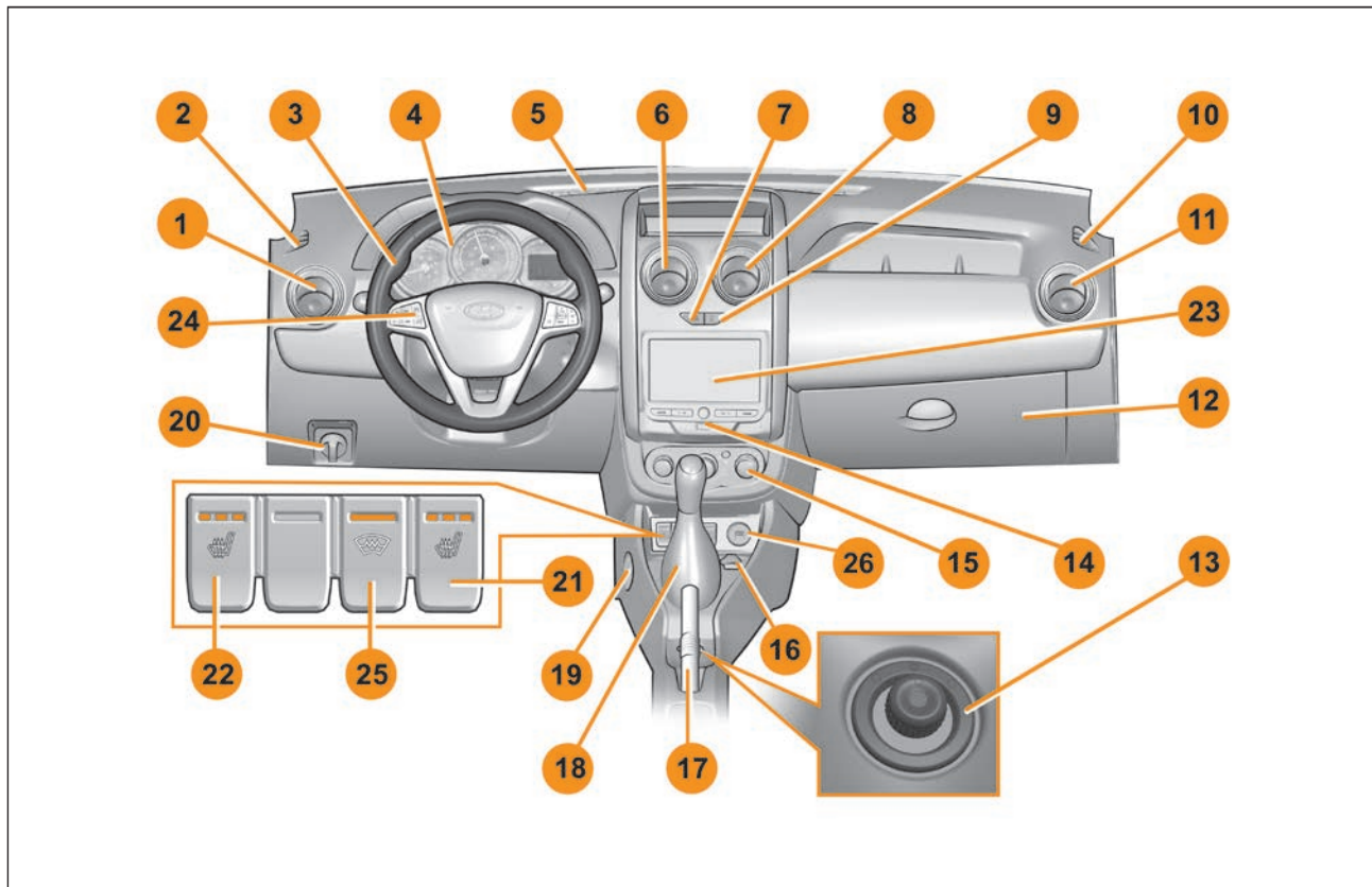
Рис. 3.1.2. Панель приборов среднего и верхнего уровня оснащения (в варианном исполнении)
